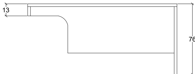
TOPO E ELEVAÇÃO MESA ESC 1:25
