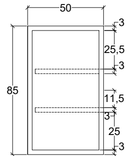
CORTE ESC 1:25
