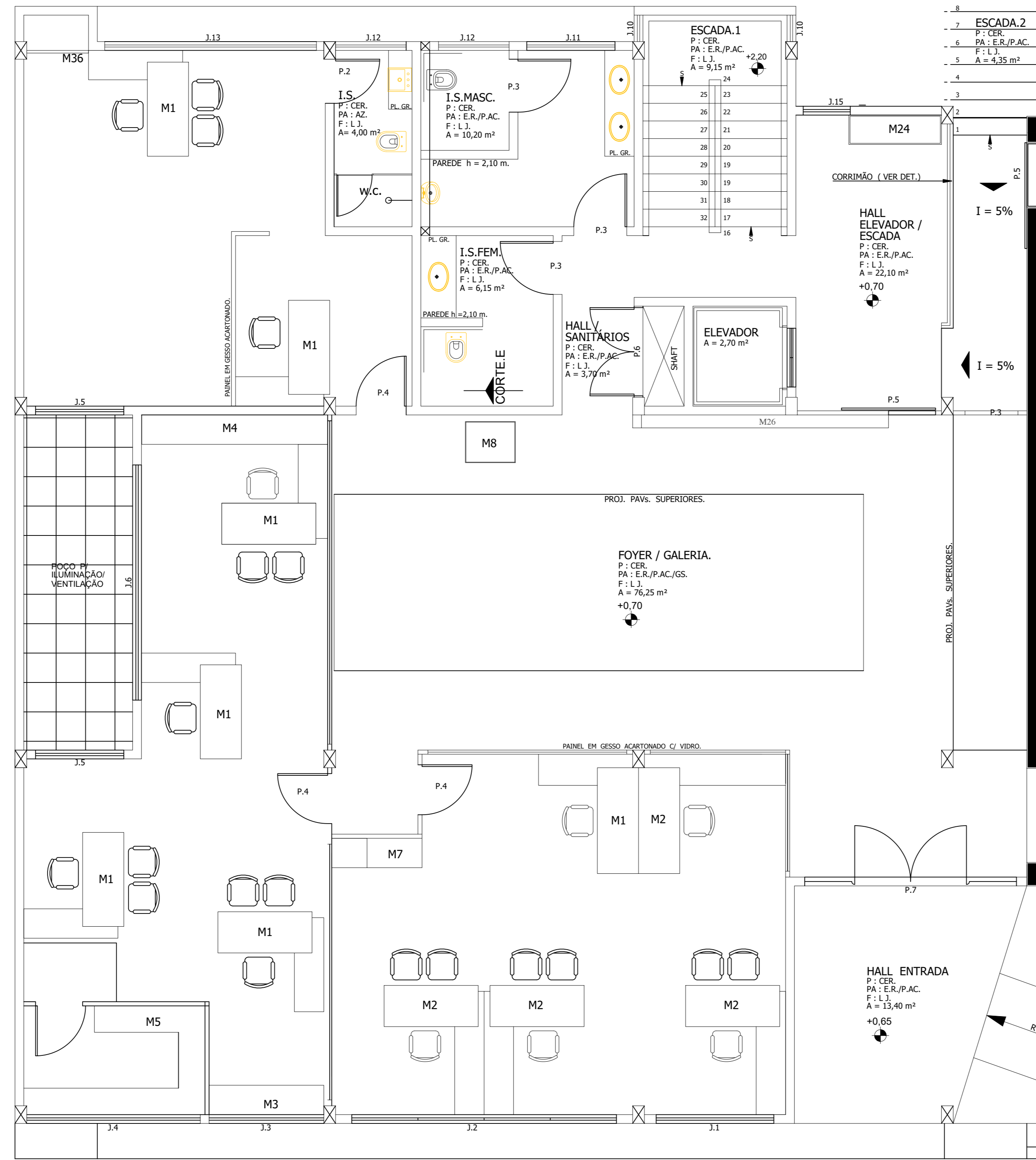
PLANTA DE LAYOUT PAVIMENTO TÉRREO ESC 1:50
