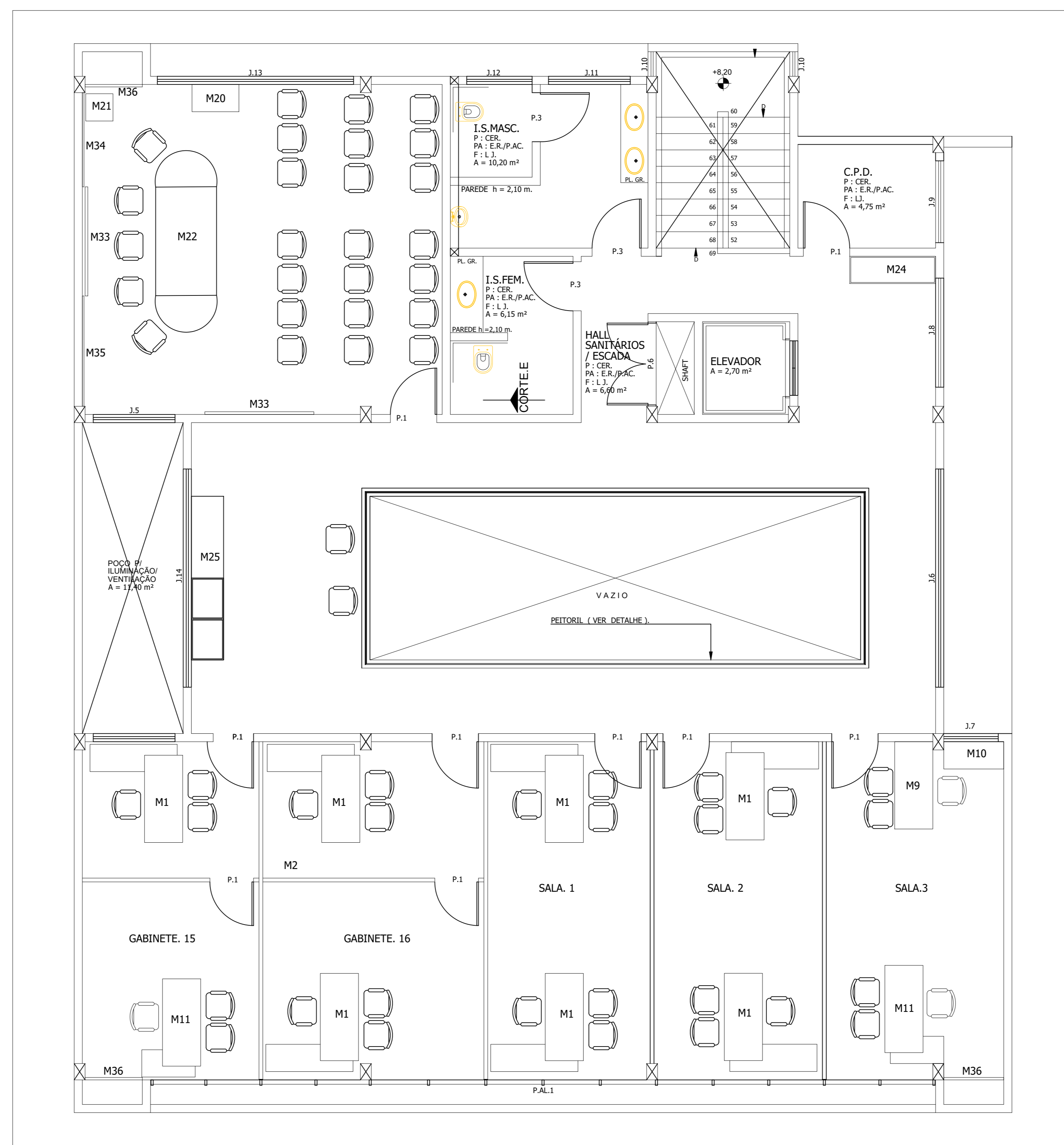
PLANTA DE LAYOUT 3º PAVIMENTO ESC 1:50
