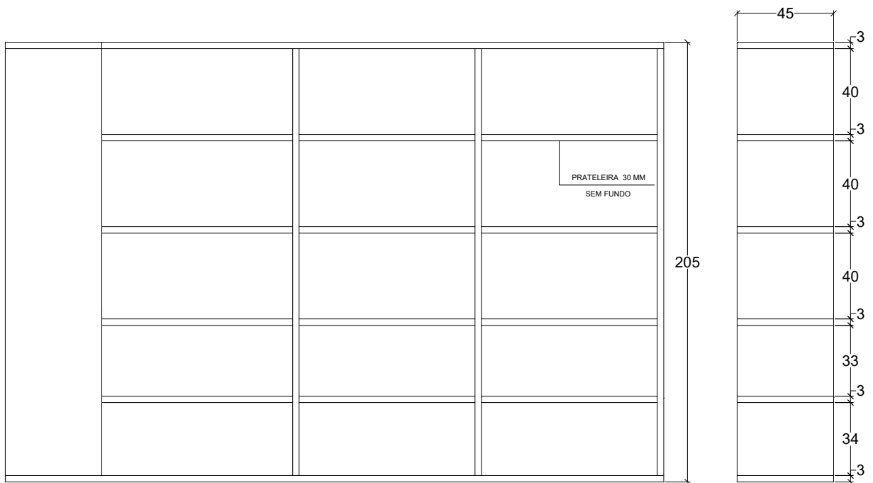
ELEVAÇÃO ESC 1:25
