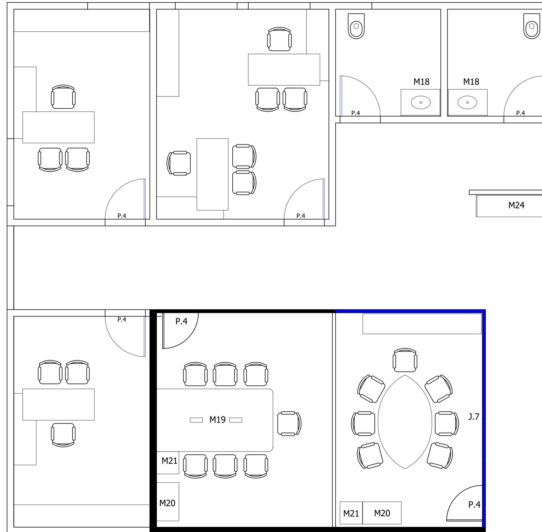
PLANTA BAIXA - 1º PAVIMENTO PRÉDIO ANEXO ESC 1:50
