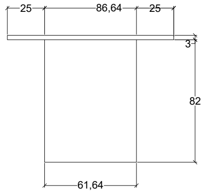
CORTE ESC 1:25
