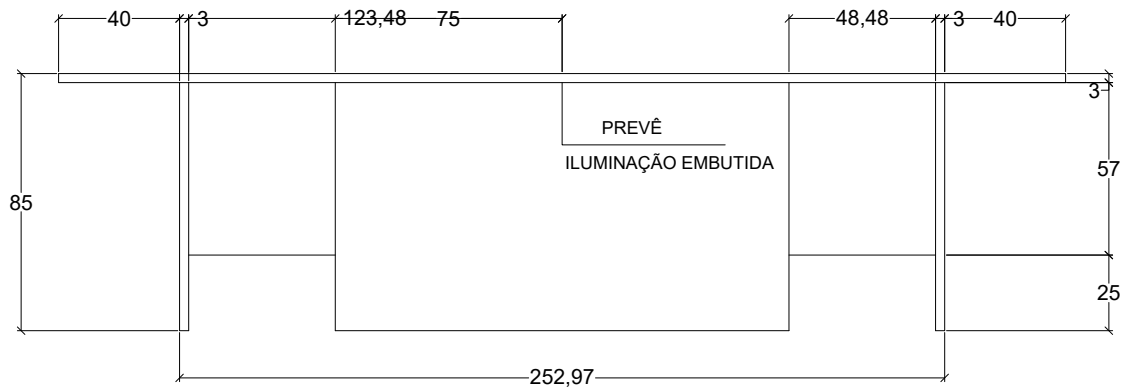
ELEVAÇÃO ESC 1:25
